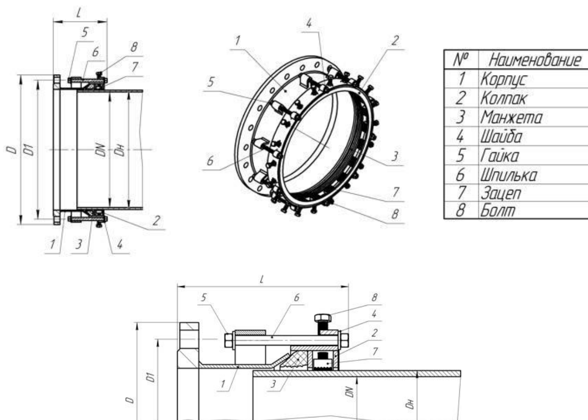
Рис. 1 Устройство муфты.
